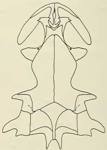
D. Reicheltia halsteadii (skull length 41 mm)
